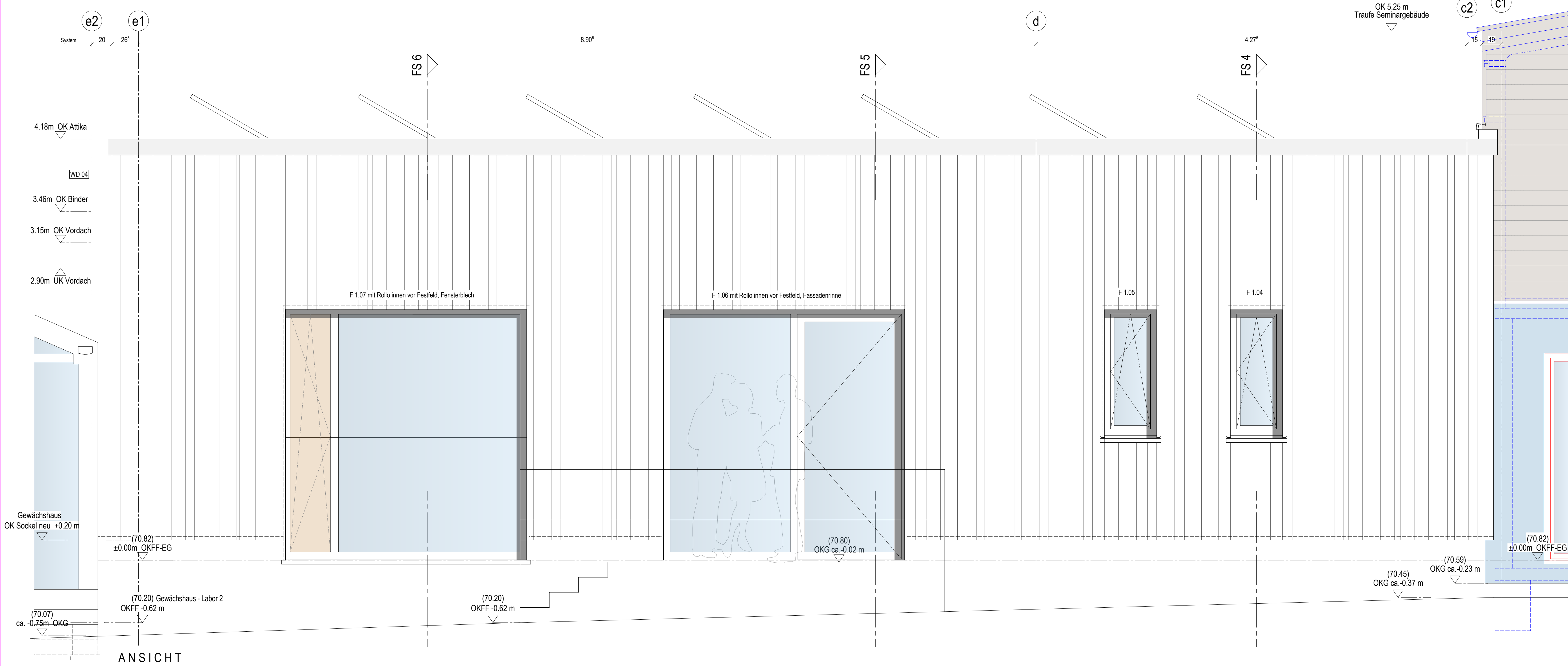
ANSICHT
