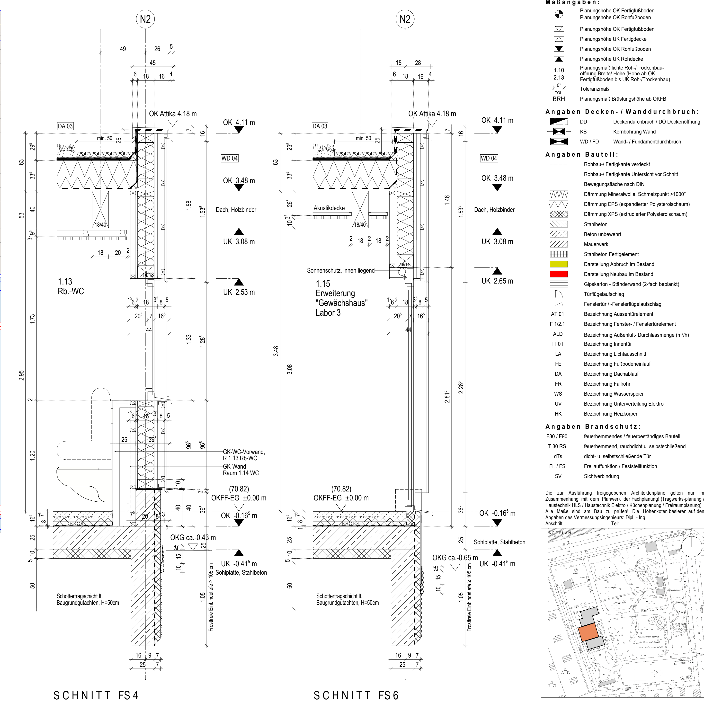
SCHNITT FS4
